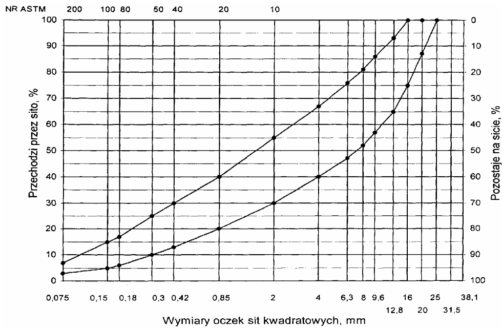
Rys. 8. Krzywe graniczne uziarnienia mieszanki mineralnej BA od 0 do 20 mm do podbudowy dla drogi o obciążeniu ruchem KR2
