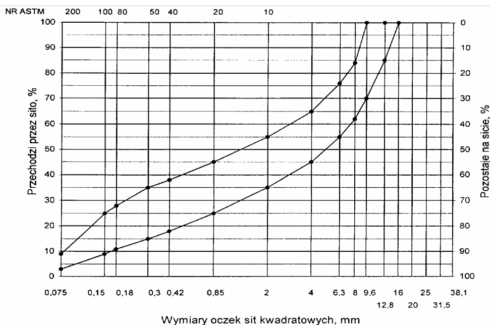
Rys. 10. Krzywe graniczne uziarnienia mieszanki mineralnej BA od 0 do 12,8 mm do podbudowy dla drogi o obciążeniu ruchem KR2
