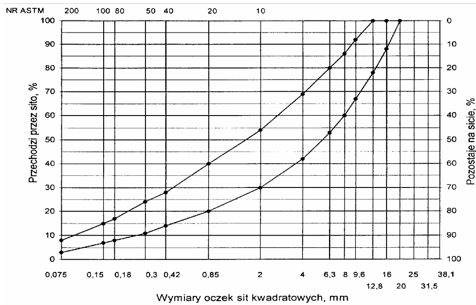
Rys. 8. Krzywe graniczne uziarnienia mieszanki mineralnej BA od 0 do 20 mm do podbudowy dla drogi o obciążeniu ruchem KR2
